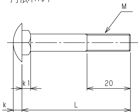
角根ボルト
